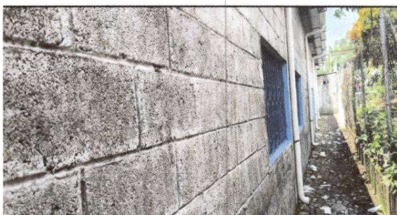
FOTO 4: Repello en muro Y Pintura en muros exteriores
